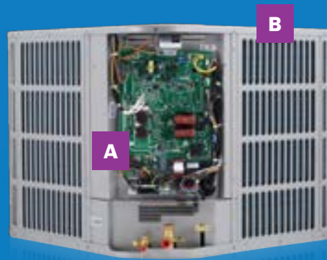
Bosch BOVB18
