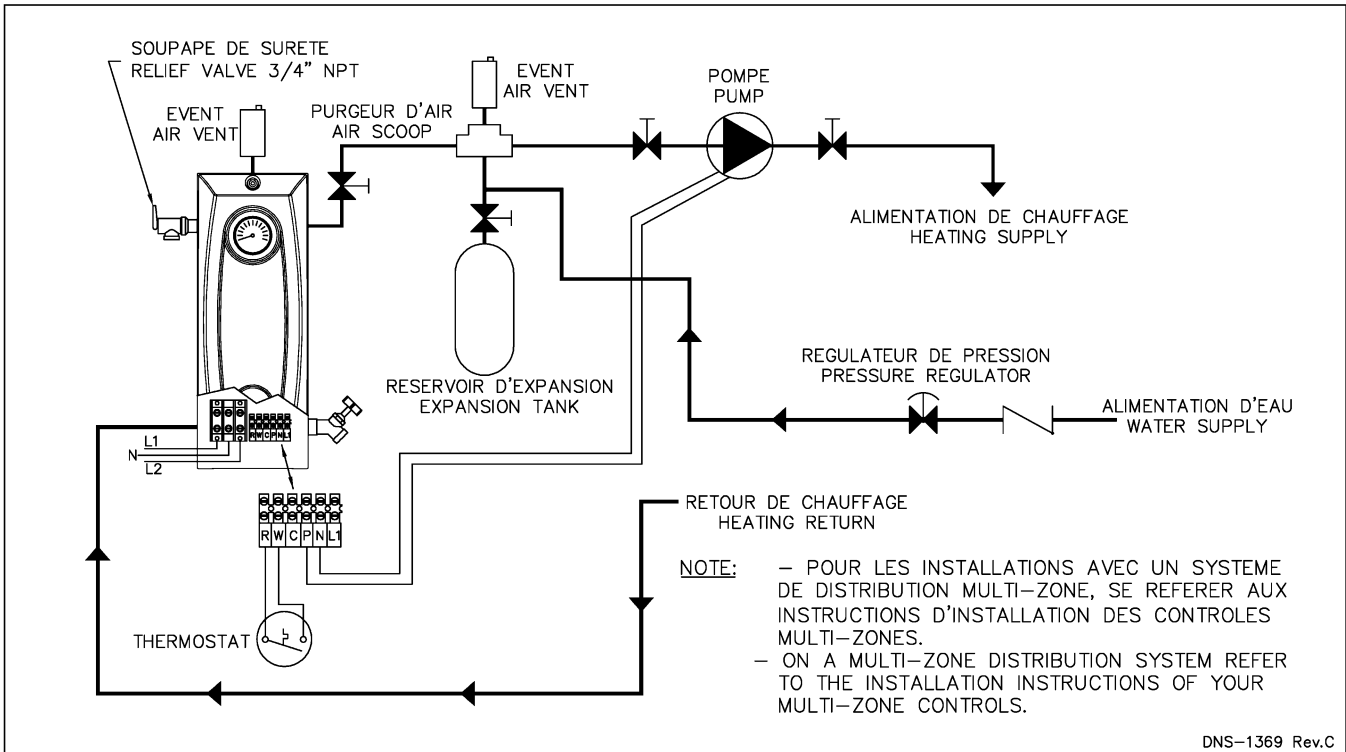
Figure 4 : Schéma type d'une installation à une zone
