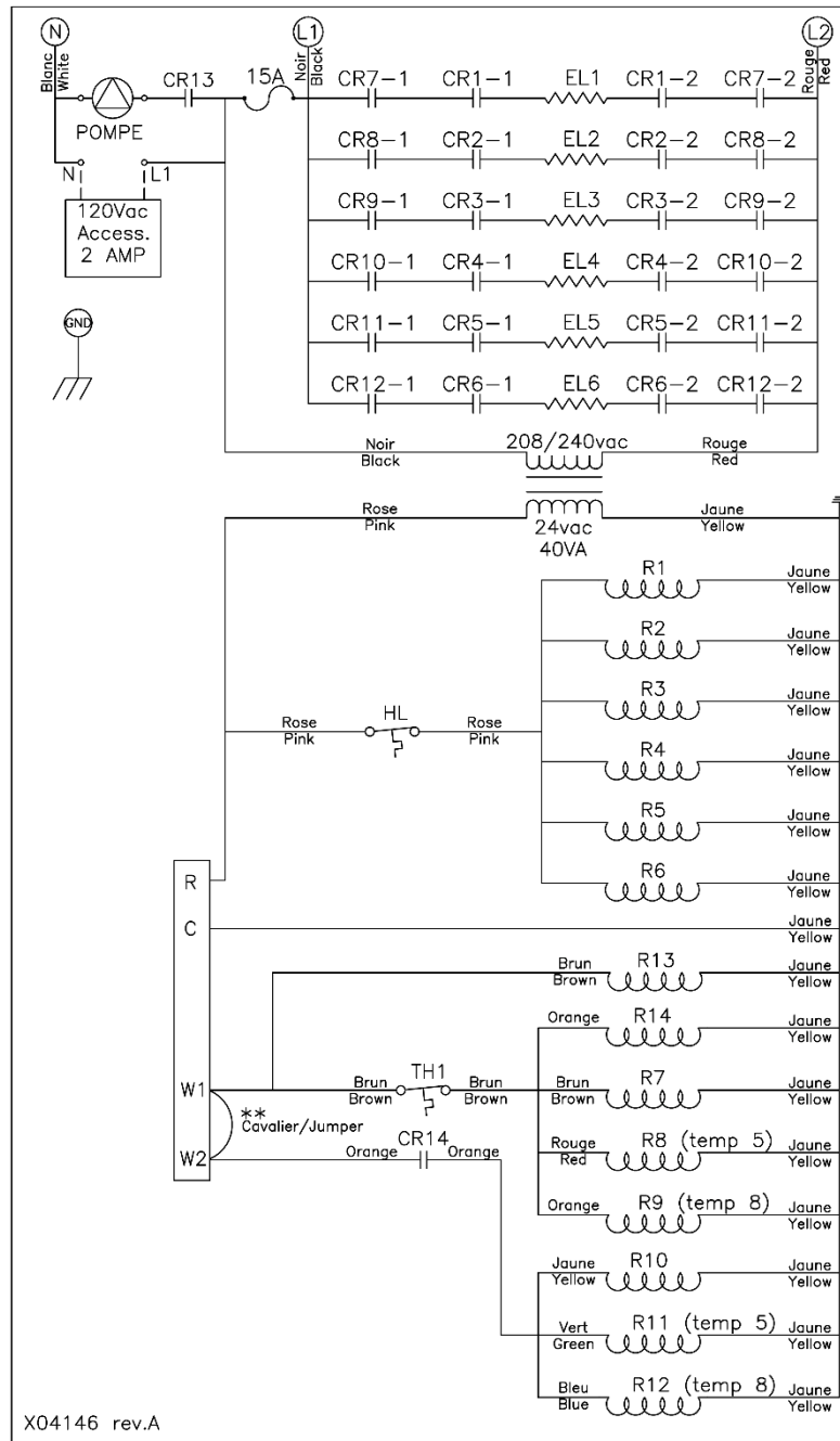
Figure 7 : Diagramme électrique
