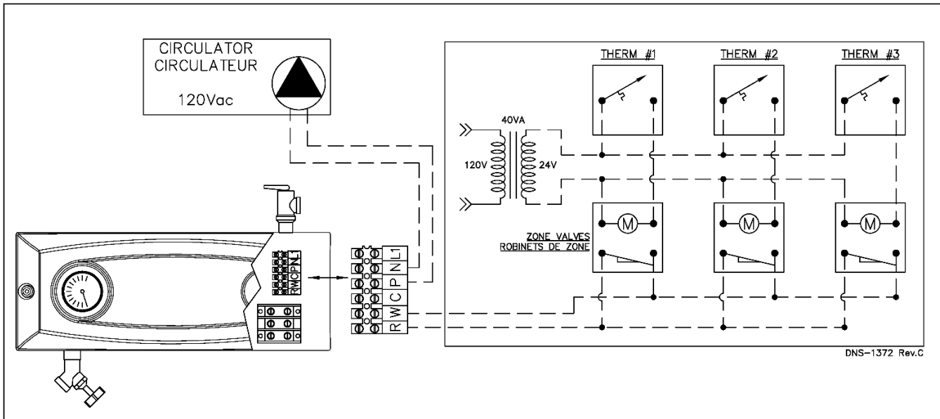
Figure 6 : Diagramme multizone avec valves motorisées
