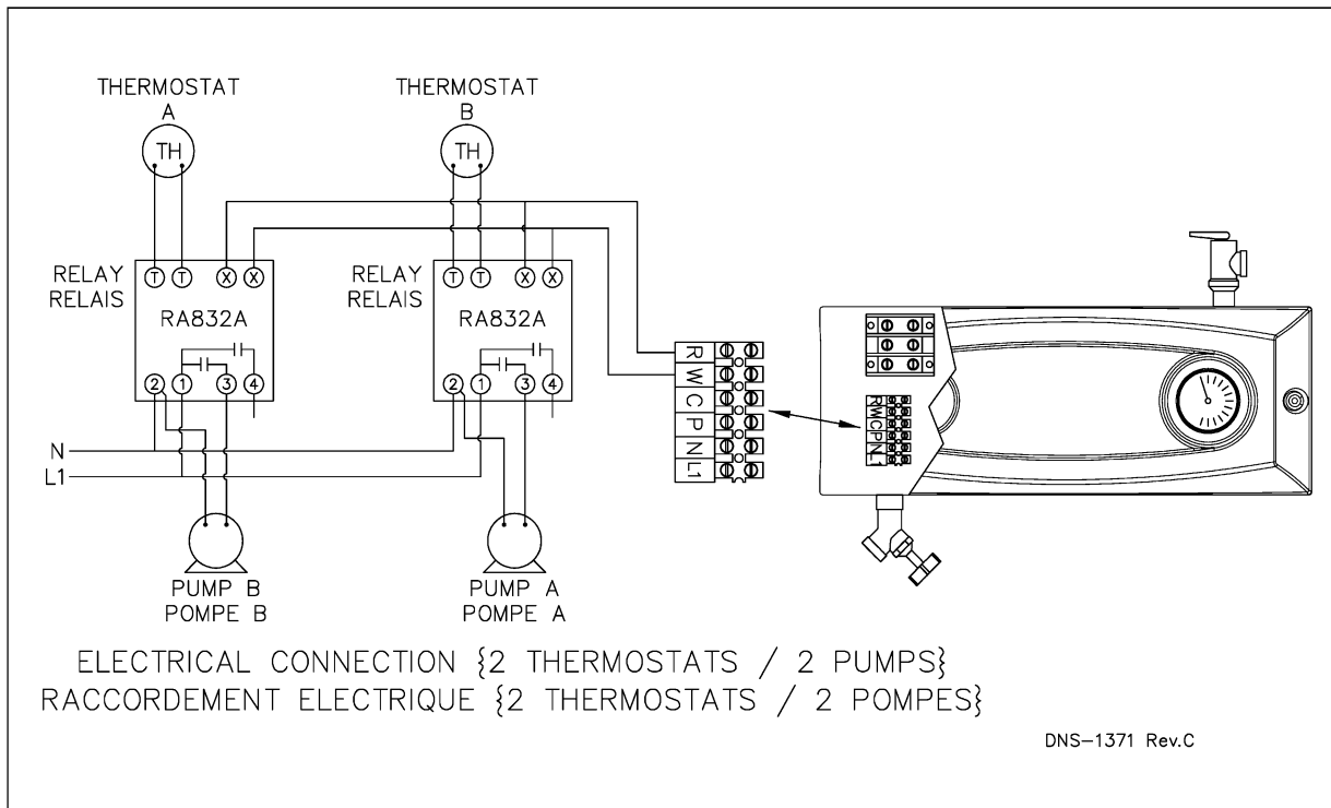
Figure 5 : Diagramme multizone avec plus d'un circulateur
